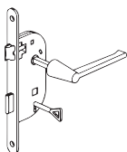
Pêne dormant 1/2 tour (PDDT)
